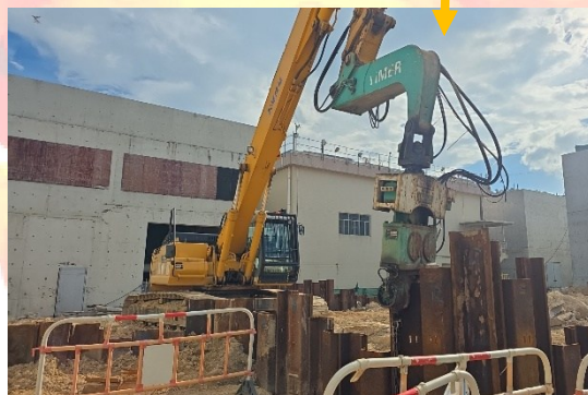
Sheet piling works for Sludge Centrifuge House in Progress 污泥離心機大樓的地基板樁工程正在進行中
